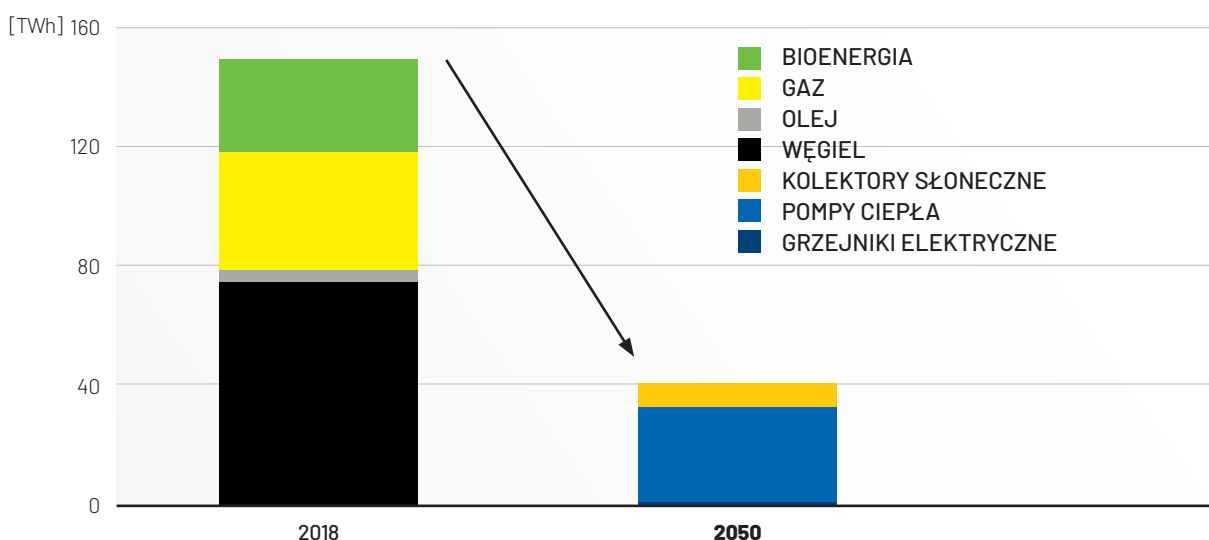
RYS. 3. ROCZNE ZUŻYCIE CIEPŁA ORAZ ŹRÓDŁA W OGRZEWANIU INDYWIDUALNYM W BUDYNKACH
